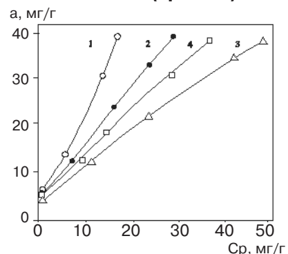
Рисунок 1 Ізотерми адсорбції фенолу сорбентами за тривалості процесу 6 год: АУВМ-66 (крива 1), АУВМ-41 (крива 2), "Бусофіт" (крива 3), АУВМ-25 (крива 4)
